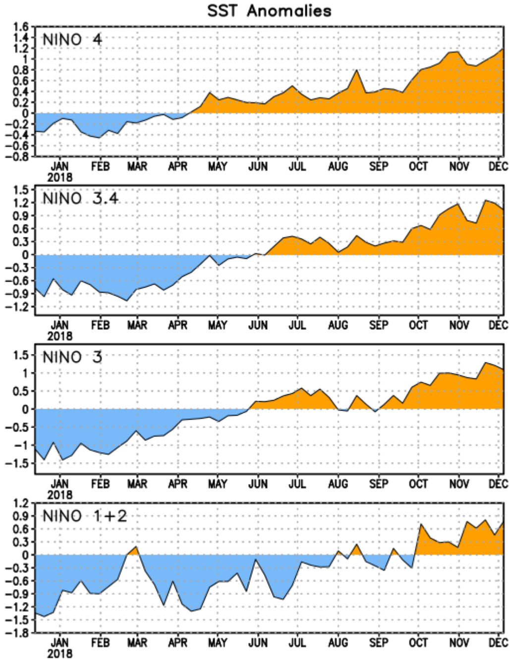
Figura 2. Series de Tiempo de las anomalías (en °C) de temperaturas de la superficie del océano (SST, por sus siglas en inglés) en un área promediada en las regiones de El Niño [Niño-1+2 (0°-10°S, 90°W-80°W), Niño-3 (5°N-5°S, 150°W-90°W), Niño-3.4 (5°N-5°S, 170°W-120°W), Niño-4 (5°N-5°S, 150°W-160°E)]. Las anomalías de SST son variaciones de los promedios semanales del período base de 1981-2010.
