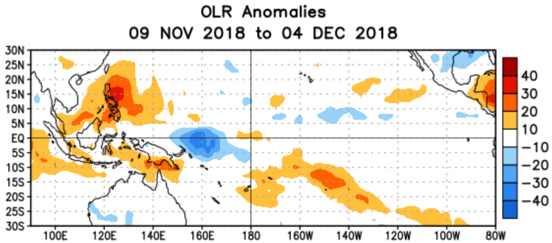
Figura 5. Anomalías promedio de la radiación de onda larga emitida (OLR, por sus siglas en inglés) ( W/m^2 ) durante el período del 9 de noviembre al 4 de diciembre de 2018. Las anomalías de OLR se calculan como desviaciones de los penta-promedios del período base de 1981-2010.
