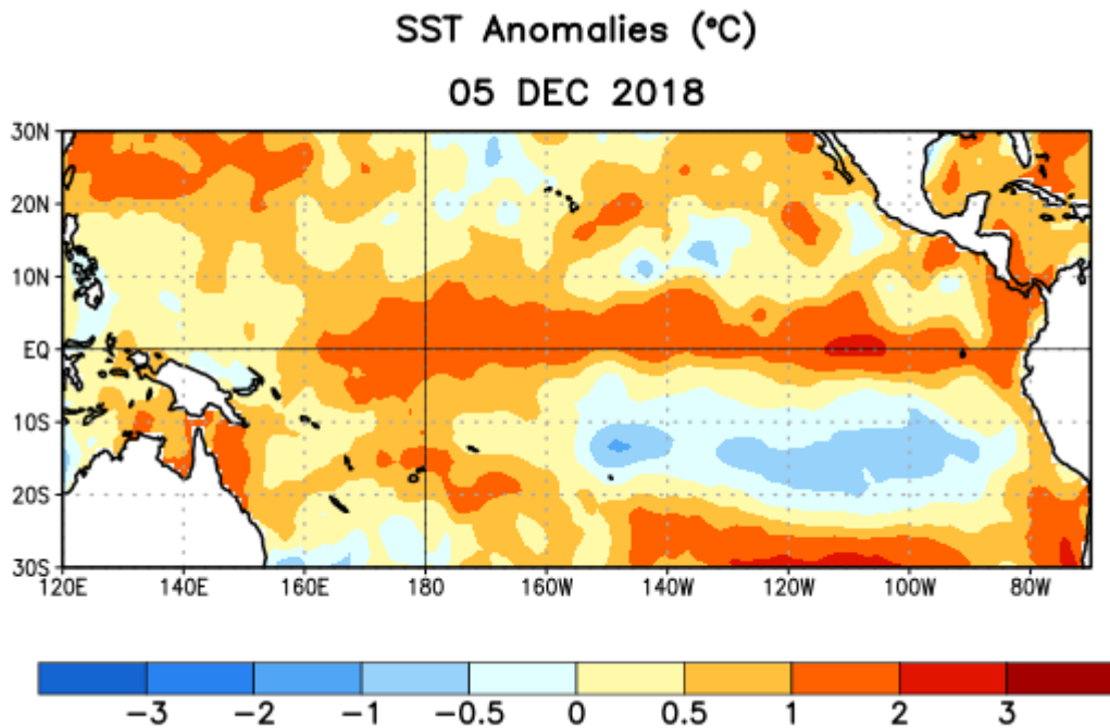
Figura 1. Anomalías (°C) promedio de la temperatura de la superficie del océano (SST, por sus siglas en inglés) para la semana centrada el 5 de diciembre de 2018. Las anomalías son calculadas utilizando como referencia los periodos promedio semanales de 1981-2010.
